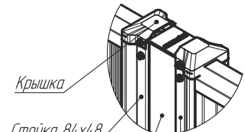
Стойка 84x4,8
